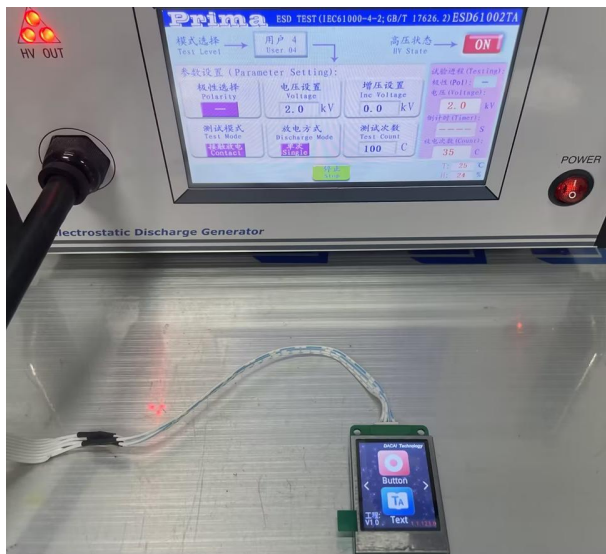
图 5-2 ESD 测试图
